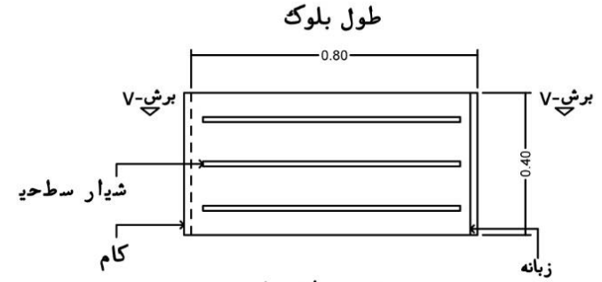
تصویر از جلو
