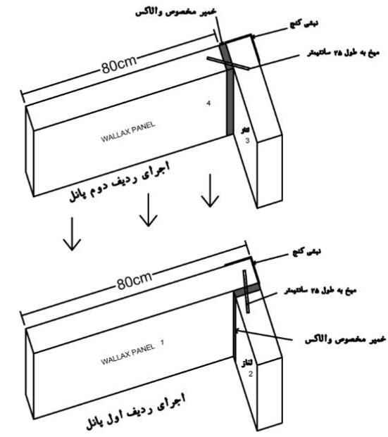
جزئیات اجرای اتصال کنج در والاکس با نبشی
