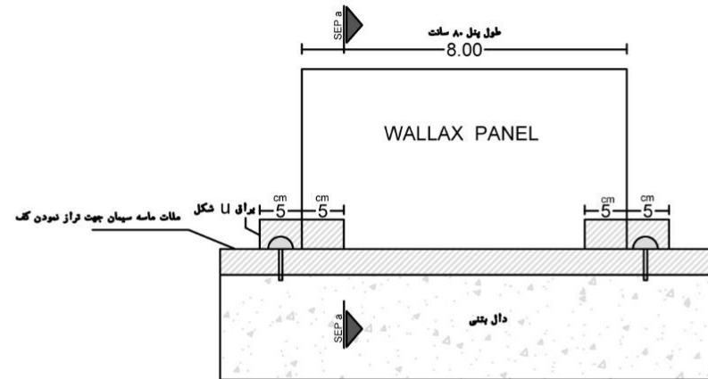
جزئیات اتصال دیوار به کف
