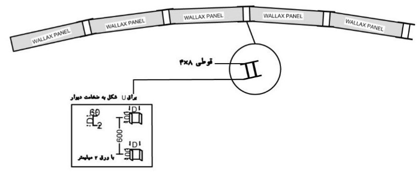
جزئیات اجرای دیوار قوسدار با پانل ها
