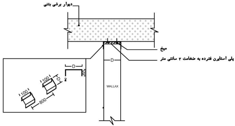
جزئیات اتصال دیوار به سقف
