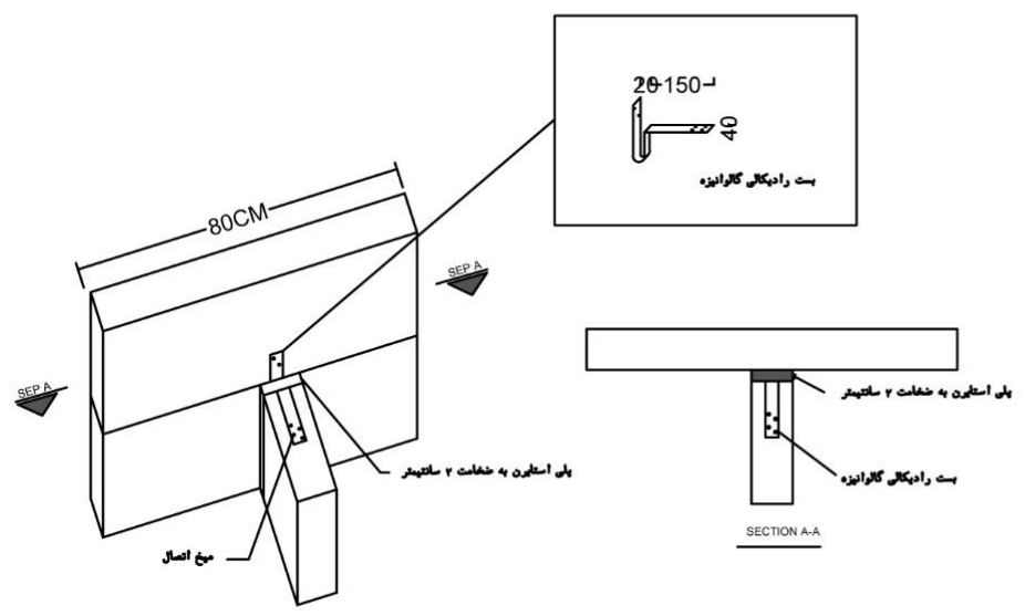
جزئیات اتصال دیوار به دیوار میانی
