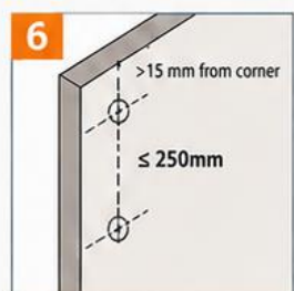
فاصله پیچ‌کاری
