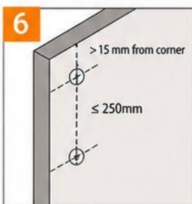
فاصله پیچکاری
